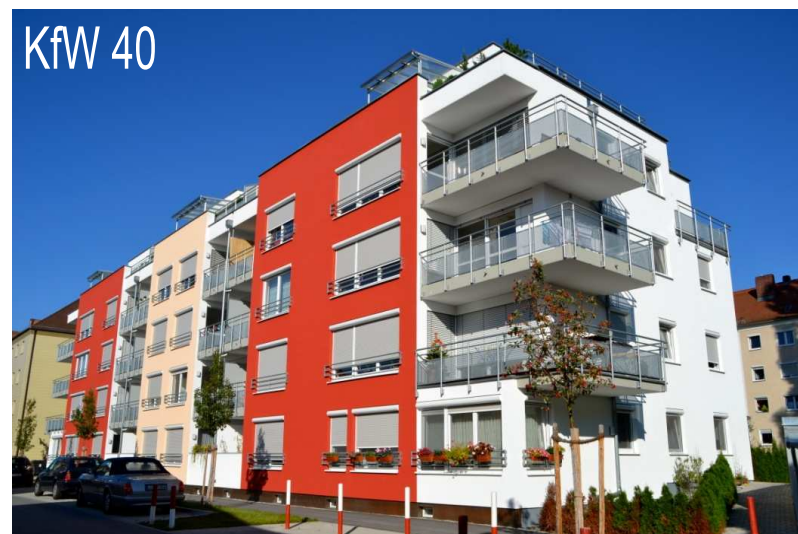
Wohnanlage Lehbühlstraße, Landshut MFH mit 27 Wohnungen, Fertigstellung 2009/2010 BHKW, Grundwasserwärmepumpe Endenergiebedarf 13,7 kWh/(m 2 a)
